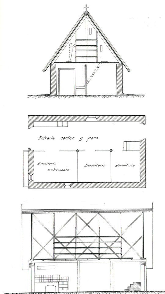
Figura 6.2. Sección, planta y alzado barraca (Gosalvez, V. [1915]1998, 21)
