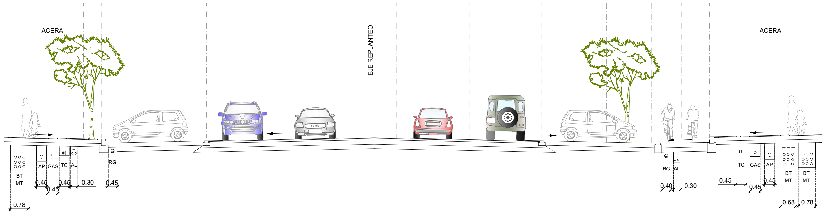
SECCIÓN 4
