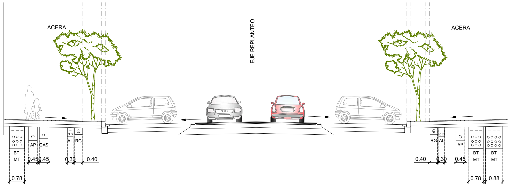
SECCIÓN 3
